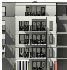
Achtergevel 1|500
